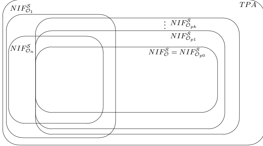
Fig. 1. NIF Hierarchy
